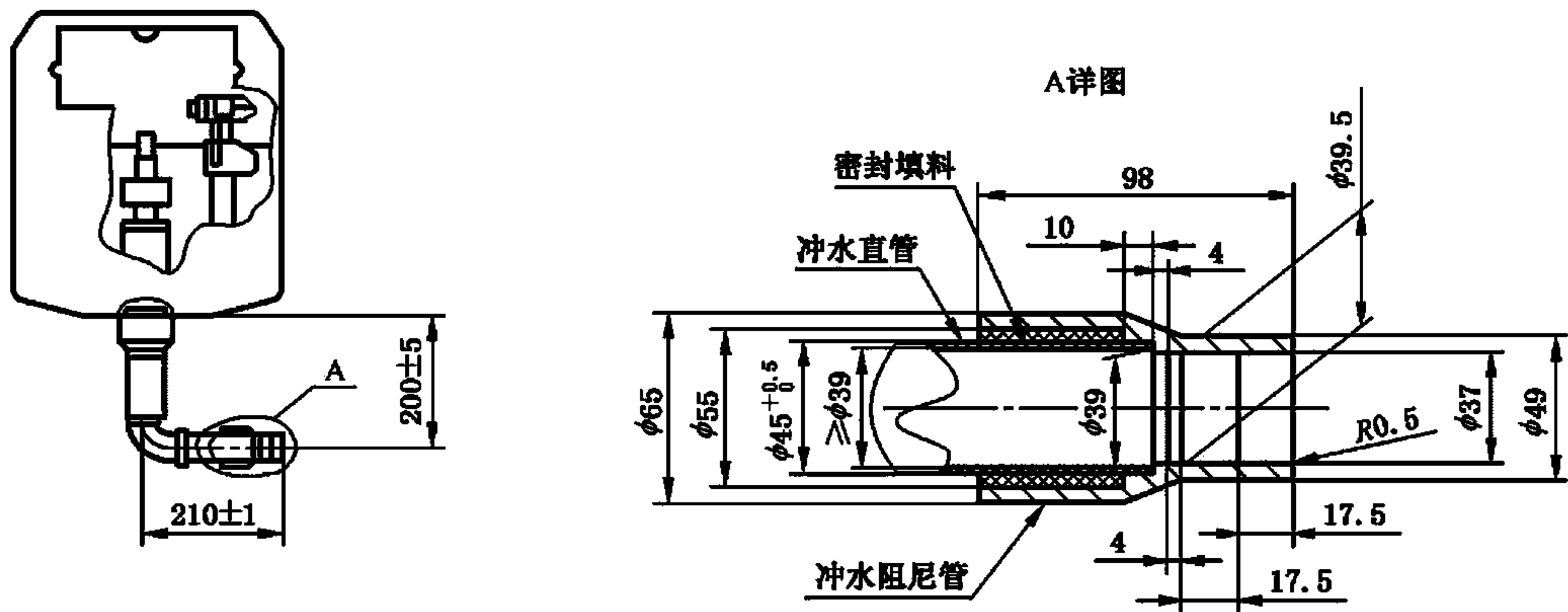
图 4 水箱冲水直管和阻尼管安装示意图
