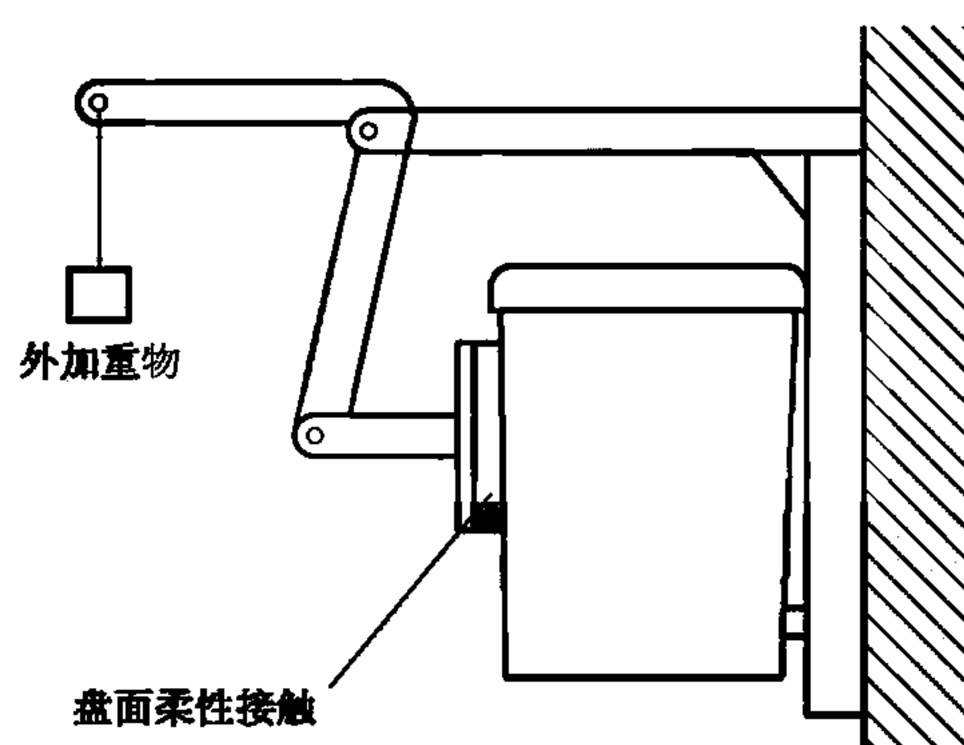
图 F.1 水箱前推力试验示意图
